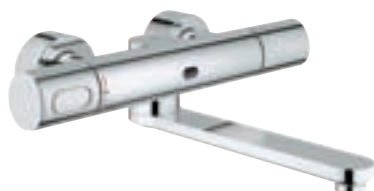
36 332 000 Infračervená, elektronická nástěnná umyvadlová baterie s termostatickým ovládáním teploty dosah 287 mm
